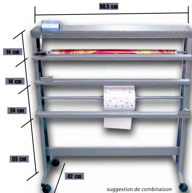
CELLOCOUPE09 SUPPORT BOBINES DIAMÈTRE MAXI 90 MM Réf. 053740
